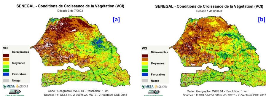
Figure 3 : Cartes du VCI de (a) la troisième décennie du mois de juillet et (b) première décennie d'août 2023
