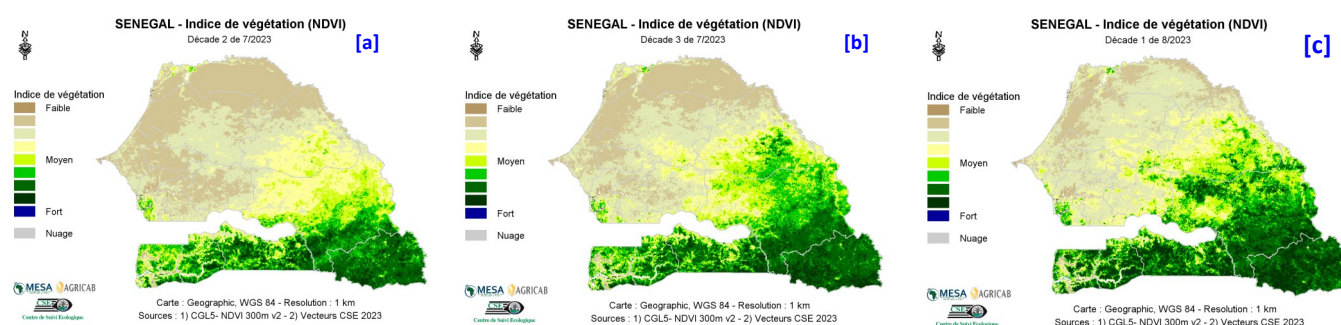
Figure 1 : Cartes du NDVI de (a) la deuxième décennie, (b) la troisième décennie du mois de juillet et (c) la première décennie du mois d'août 2023
