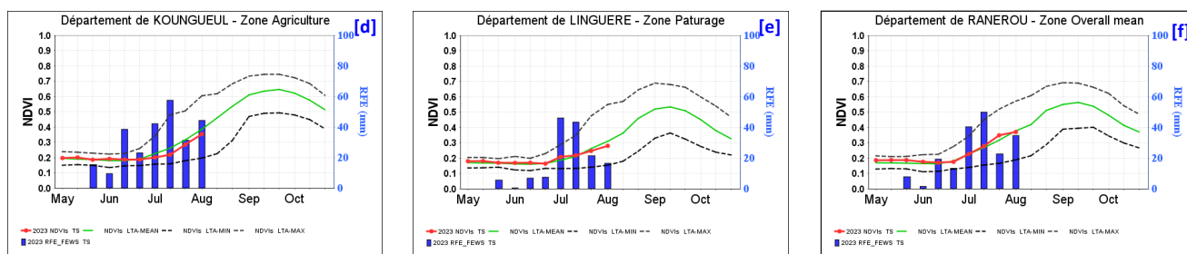
Figure 2 : Evolution du profil du NDVI dans les départements de (d) Kounghoul (zone agricole), (e) Linguère (zone pastorale) et (f) Ranérou (zone Overall mean).
