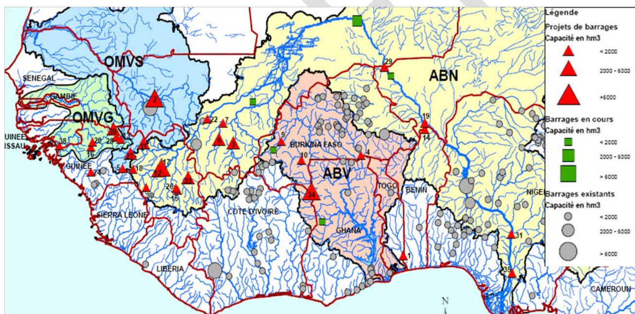
Barrages existants, en cours et en projet (CEDEAO, 2011)
